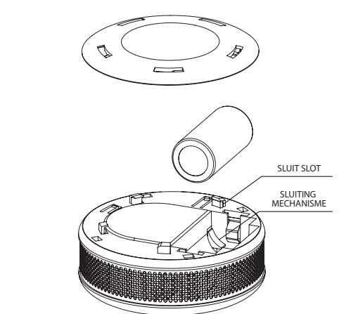
Fig. 2 - Fibaro Rook Sensor onderaanzicht zonder de batterij geïnstalleerd
